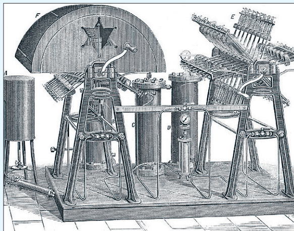
Toestel Beins voor het vullen van kogelflesjes
