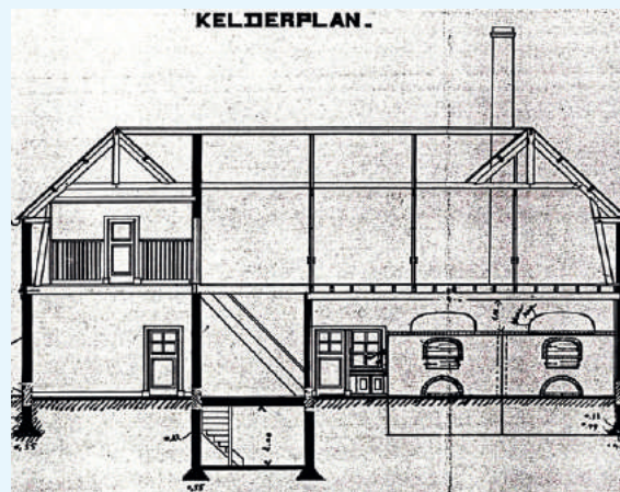
Plan voor bakkerij aan de Hamerstraat (doorsnede).
