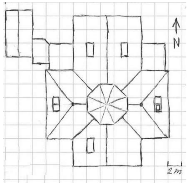
Bovenaanzicht Gen. de la Rey laan 12 en 12a (coll.HKB)
